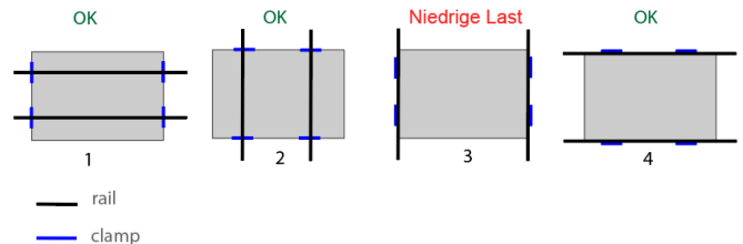
Abbildung 3: Montagekonfigurationen
